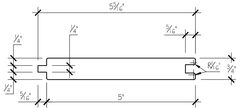
COUPE - PIN DE L'OUEST ÉCHELLE: 6"= 1'-0"
